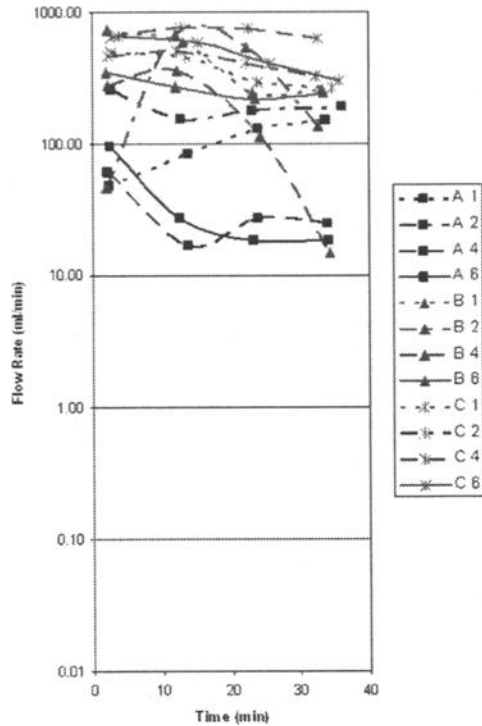
FIG. 4—Plus 3/16 confinement.
